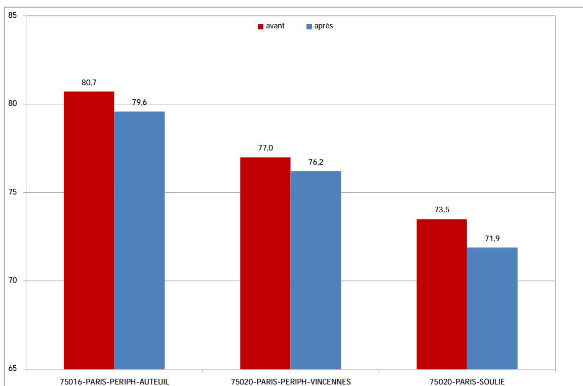
Comparaison des niveaux de bruit nocturnes (LAeq 22-6h) exprimés en dB(A) sur les stations du périphérique avant et après l'entrée en vigueur de la baisse de la vitesse limite
